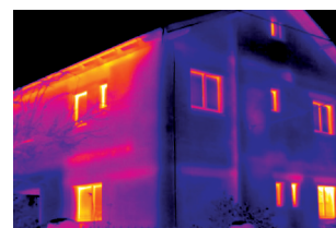
Detekcja strat ciepłych w budynkach: natychmiastowa lokalizacja mostków cieplnych
